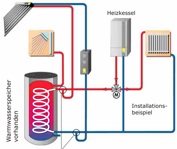
Nur diesen beiden T-Stücke werden für den Anschluss des Solarkreises benötigt. Alles andere bleibt unverändert.
